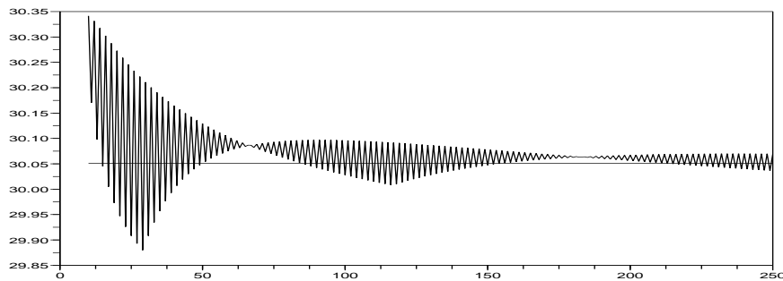
FIGURE 1 – Tracé du prix Cox, Ross et Rubinstein C_0(n) d'un Call Européen en fonction de n et de sa limite, le prix Black-Scholes. Valeur des paramètres : S_0 = 140 , \sigma = 0.40 , r = 0.05 , et K = 130
