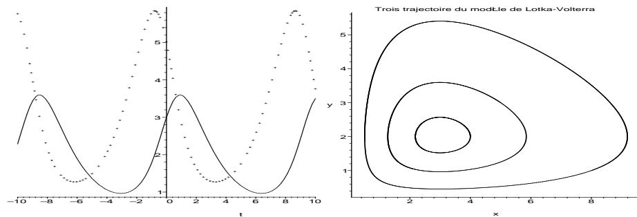
FIG. 1 – A gauche le graphe des effectifs des proies x(t) (en pointillés) et celui des prédateurs y(t) (en trait plein), dans le cas où x(0) = 5 et y(0) = 3 . A droite plusieurs trajectoires du système (2) représentées dans le plan de phase (la trajectoire du milieu est issue du point de coordonnées (x(0) = 5 ; y(0) = 3) et correspond aux deux graphes de gauche).
