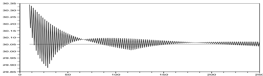
FIGURE 10.1 – Tracé du prix CRR C_0(n) d'un Call Européen en fonction de n et de sa limite, le prix BS. Valeur des paramètres : S_0 = 140 , \sigma = 0.40 , r = 0.05 , et K = 130
